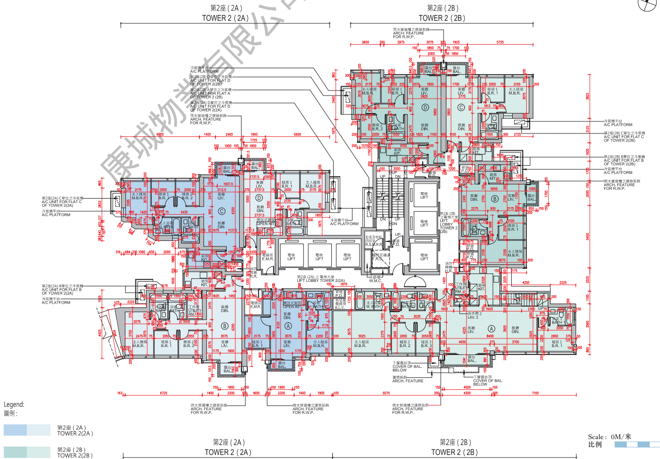
Tower 2(2A) & Tower 2(2B) 70/F Floor Plan 第2座(2A)及第2座(2B) 70樓 樓面平面圖
